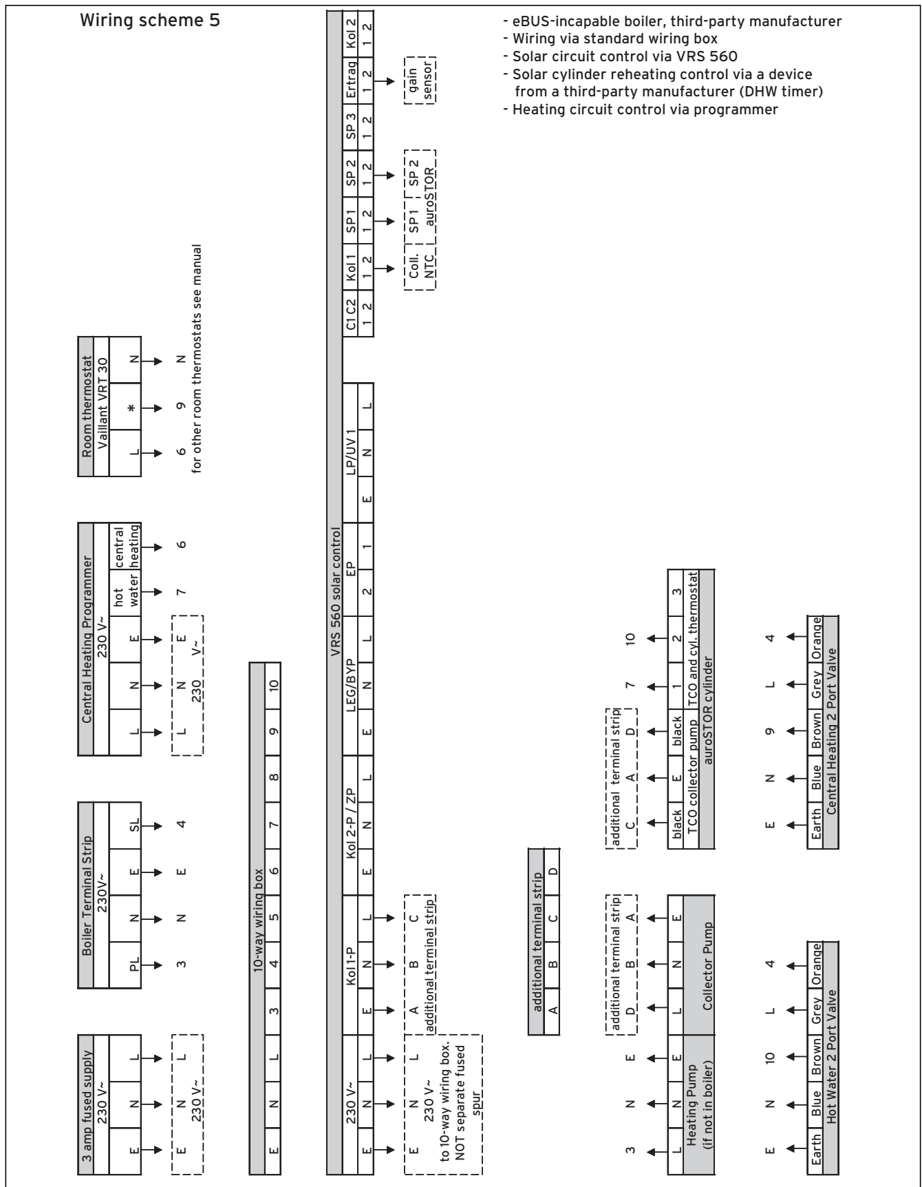
Fig. 5.37 Wiring scheme 5
