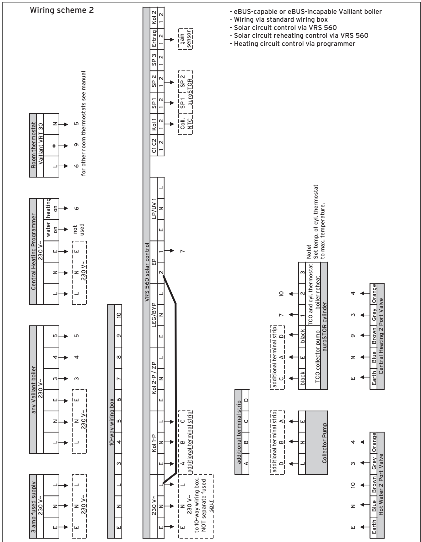
Fig. 5.28 Wiring scheme 2
