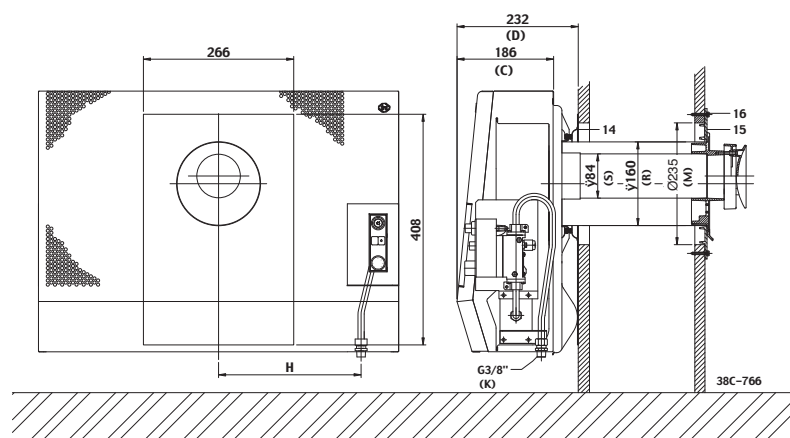
fig 10 DRU-ART 3,4
